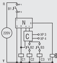
CIRCUITO DE COMANDO 220
